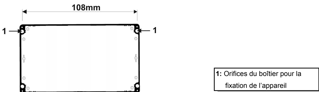
Figure 2: Emplacement des orifices de fixation (vue intérieure sans couvercle)
