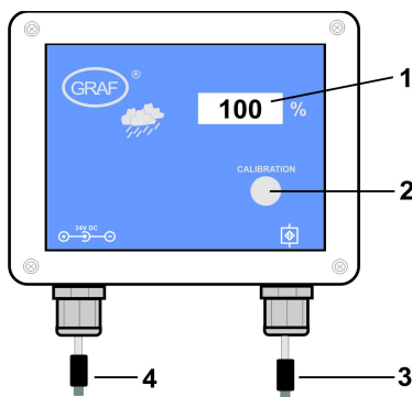
Figure 1: Aperçu de l'appareil
